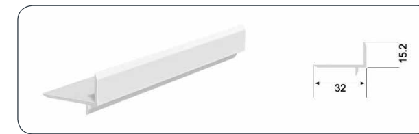
T-PROFILE
