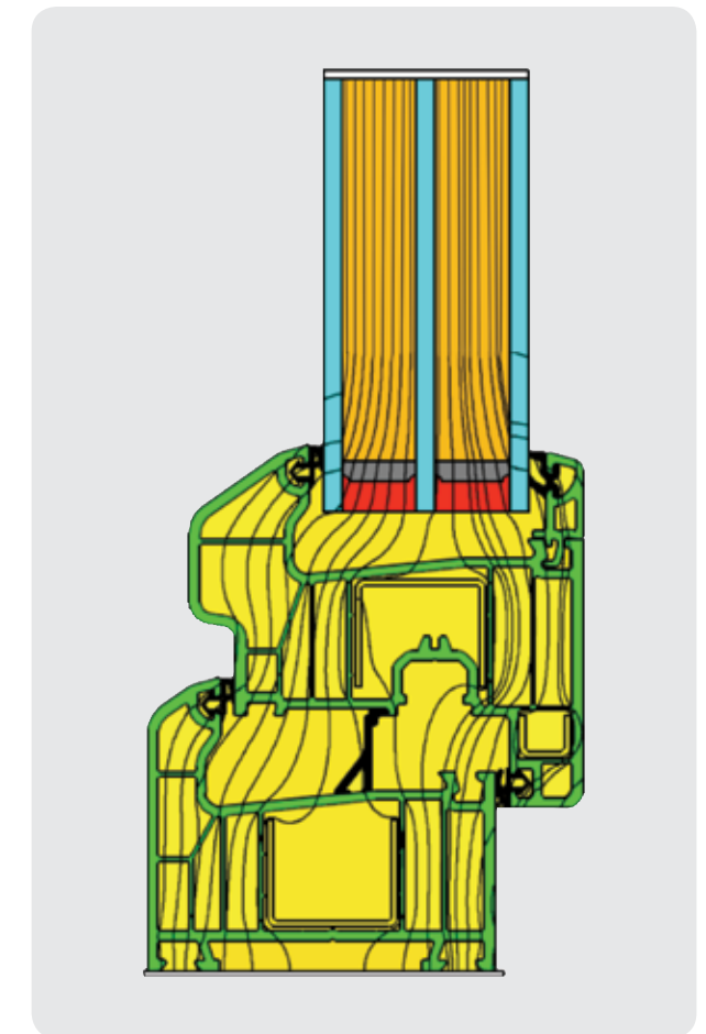
WINDOW HEAT FLOW DIAGRAM UF:1,02 W/M² °K UW: 0,94 W/M² °K
